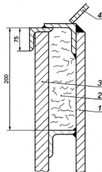
Рисунок Q.5 — Типовое исполнение теплоизоляции, закрепляемой исключительно на стенке резервуара, под выступом крыши
