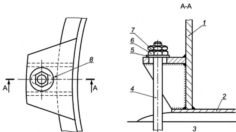
1 — стенка резервуара; 2 — днище резервуара; 3 — фундамент; 4 — анкерный болт; 5 — шайба; 6 — гайка; 7 — контргайка; 8 — отверстие в анкерном столике
