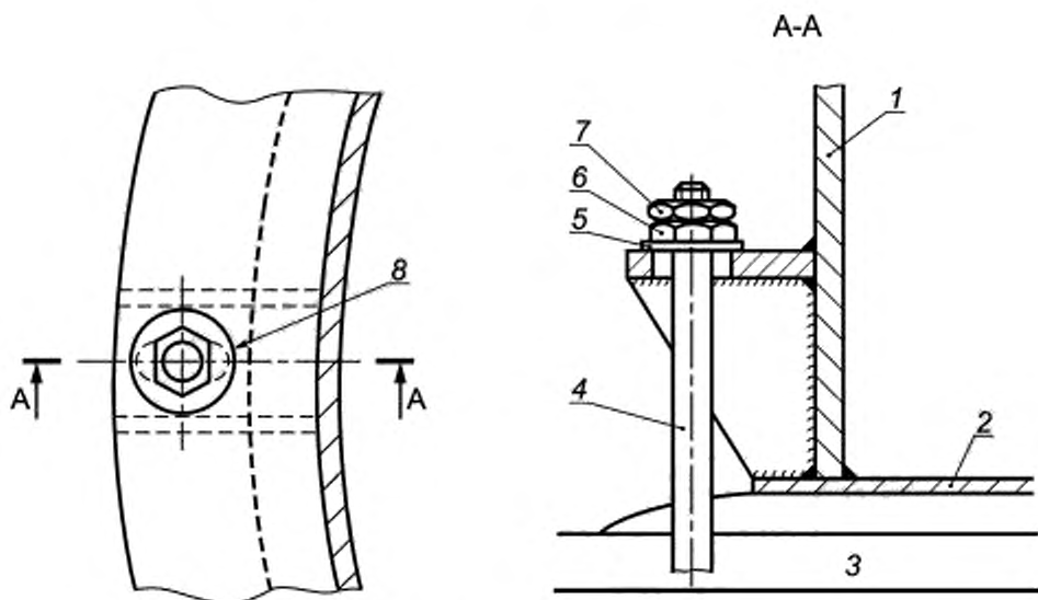
1 — стенка резервуара; 2 — днище резервуара; 3 — фундамент; 4 — анкерный болт; 5 — шайба; 6 — гайка; 7 — контргайка; 8 — отверстие в кольцевой анкерной плите
