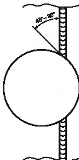
Рисунок 17 — Отверстия для патрубков, пересекающих швы стенки
