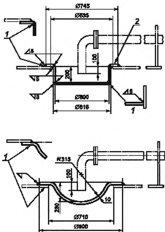
Рисунок 0.5 — Типовое исполнение зумпфов резервуаров
