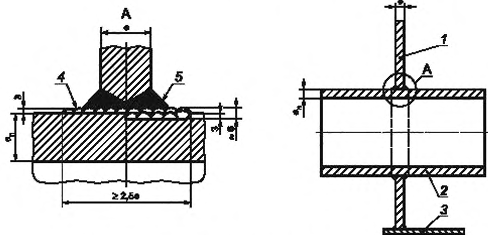
1 — лист стенки; 2 — патрубок; 3 — лист дна; 4 — наплавленный металл; 5 — указания по сварке см. в приложении N
