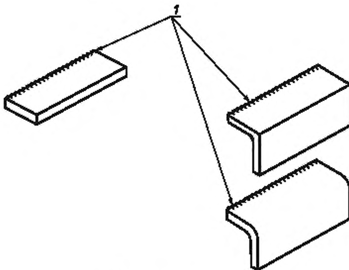
Рисунок Q.2 — Крепежные уголки и листы
