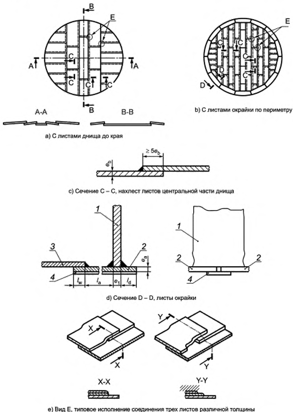
Рисунок 3 — Типовые конструкции дна резервуара
