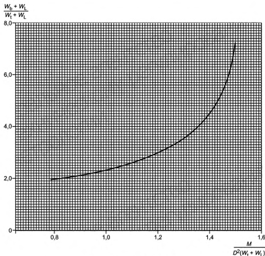
Рисунок G.4 — Усилия сжатия W_b
