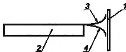
б) Пружинный первичный затвор и губчатый затвор
