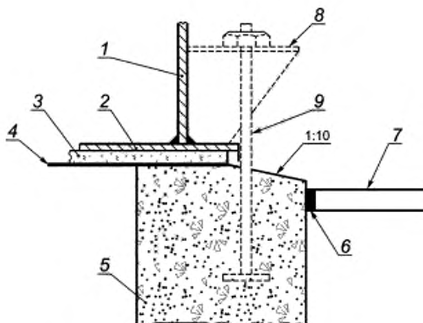
Рисунок I.1 — Грунтовая подушка
