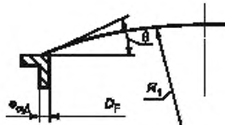
Рисунок К.2 — Сферическая крыша
