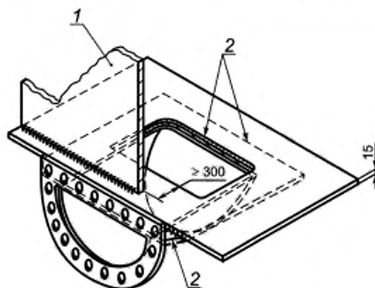
Рисунок 0.5 — Типовое исполнение зумпфов резервуаров
