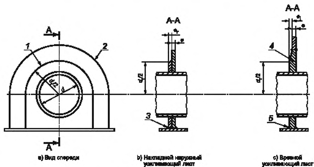
Рисунок 11, лист 1 — Усиление патрубка, расположенного около дна
