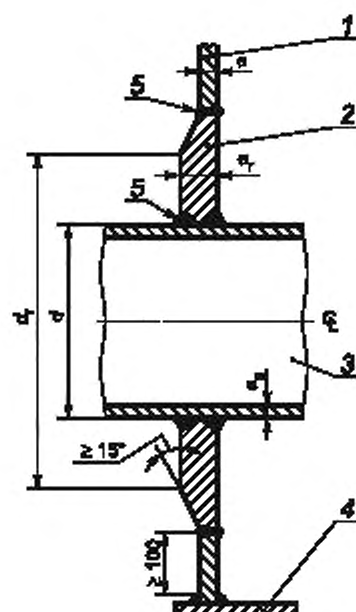
Рисунок 10 — Врезной лист в качестве элемента усиления (см. 12.1.6)
