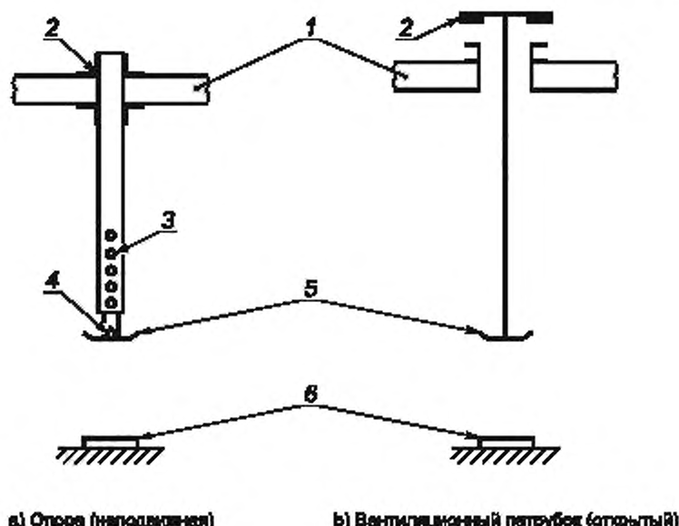
а) Опора (надувная)
