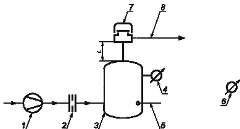
1 — устройство для подачи испытательной среды (воздуходувка или вентилятор); 2 — калиброванное устройство для измерения скорости потока; 3 — испытательный резервуар; 4 — калиброванное устройство для измерения давления и вакуума; 5 — устройство для измерения температуры; 6 — барометр — устройство для измерения атмосферного давления; 7 — испытуемый клапан; 8 — выпускная труба, если установлена, L — длина присоединительной трубы (прямого патрубка)
