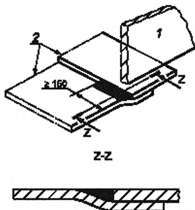
1 — лист стенки; 2 — лист днища в краевой части
