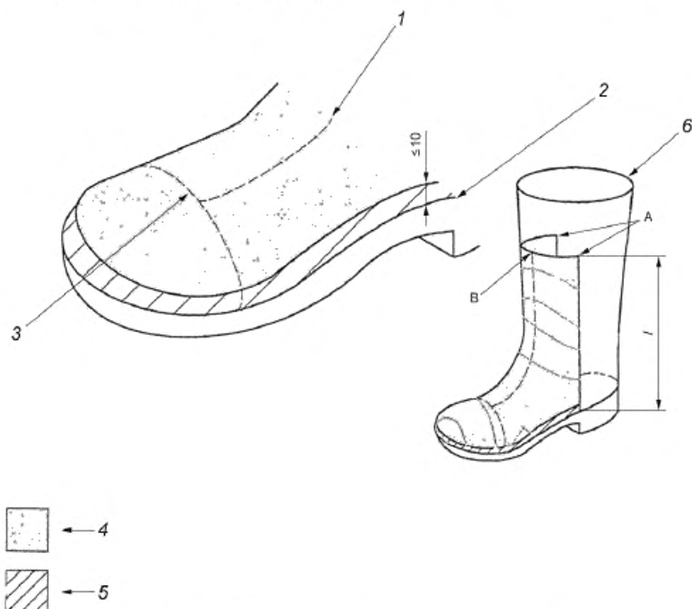
1 — геометрическая ось обуви; 2 — линия кромки; 3 — спинка носка; 4 — защитная область; 5 — дополнительная защитная область для обуви уровней защиты 3 и 4; 6 — верхний край верха обуви
