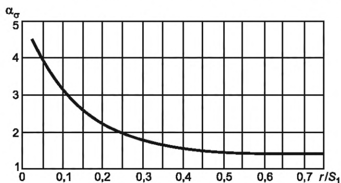
Рисунок 4 — График \alpha_\sigma
