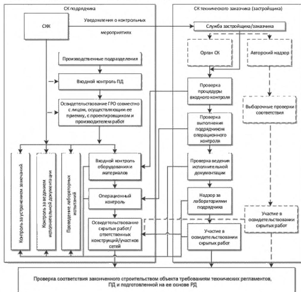
Рисунок 1 — Схема осуществления СК
