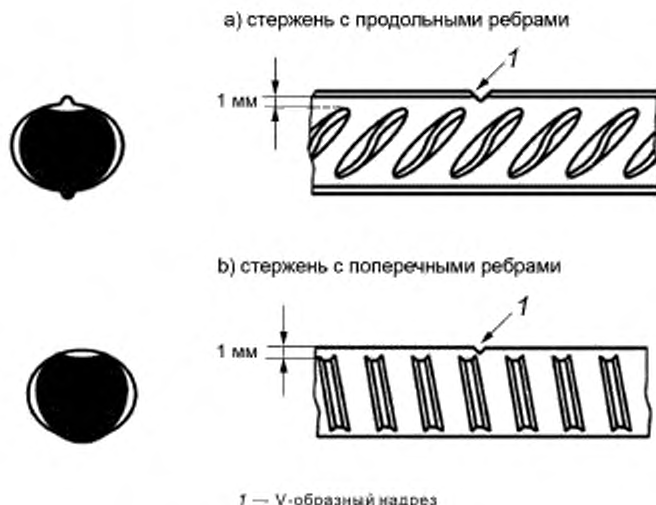
Рисунок А.1 — Надрез на арматурном стержне
