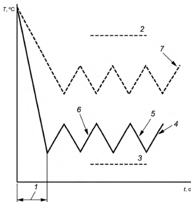
1 — период охлаждения; 2 — заданный уровень предупреждения (высокая температура); 3 — заданный уровень предупреждения (низкая температура); 4 — контролируемый датчик; 5 — обогрев выключен; 6 — обогрев включен; 7 — другой датчик
