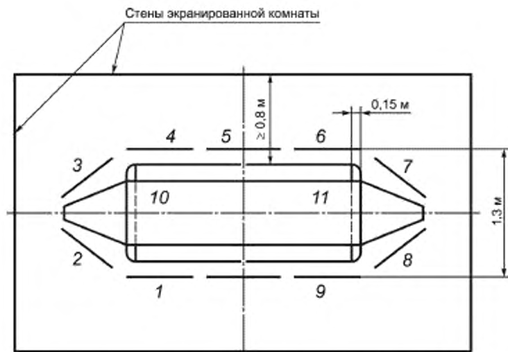
Рисунок 5 — Пример схемы ТЕМ-устройства на базе открытой полосковой линии в комбинации с поглощающими панелями внутри экранированной комнаты размерами 3 x 3,5 м
