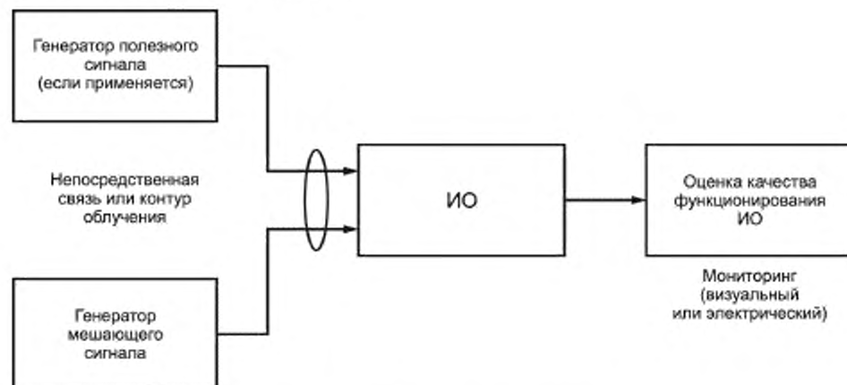
Рисунок 1 — Основная концепция измерения помехоустойчивости
