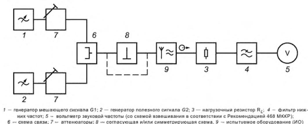
Рисунок 3 — Измерительная установка для измерения помехоустойчивости на входе приемников звукового вещания
