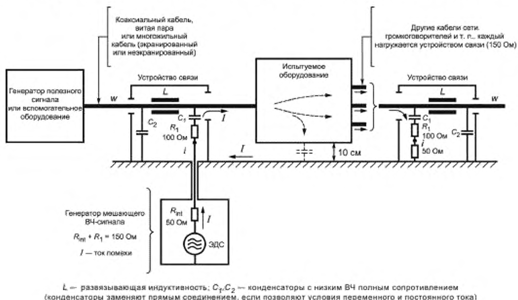
Рисунок 2 — Общий принцип метода инжекции тока
