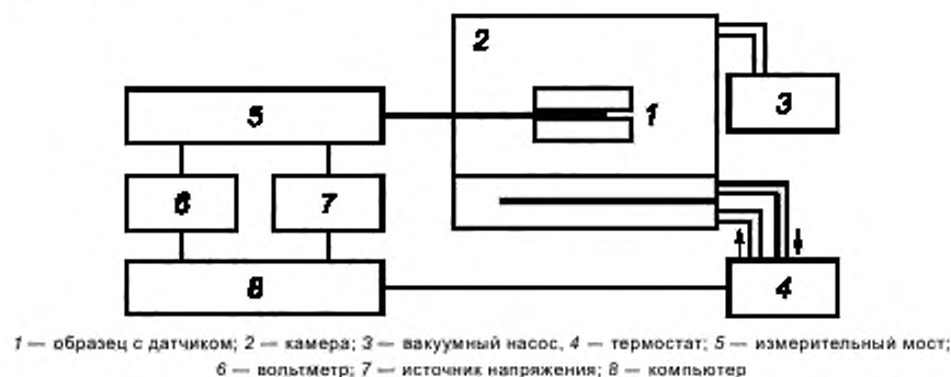
Рисунок 1 — Схема типового испытательного прибора
