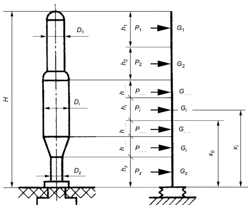
Рисунок 1 — Расчетная схема аппарата колонного типа
