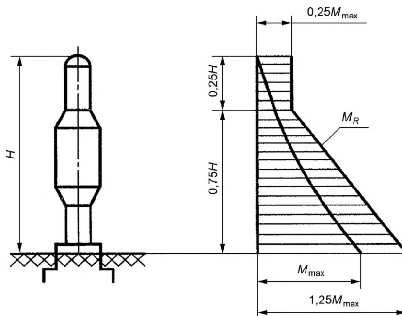
Рисунок 3 — Эпюра для определения изгибающего момента M_{\max}
