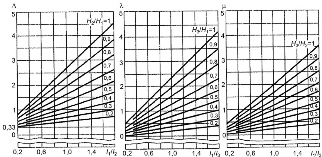
Рисунок А.1 — Коэффициенты \Delta , \lambda , \mu
