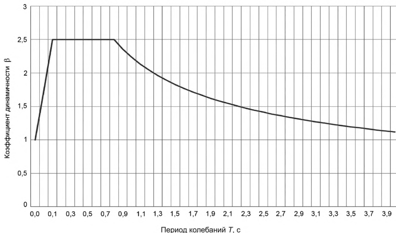
Рисунок 2 — Обобщенный спектр ответа
