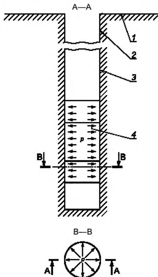
1 — поверхность земли; 2 — грунт; 3 — карман; 4 — расширяющийся зонд — прессиометр; p — приложенное давление А—А — осевое сечение; В—В — поперечное сечение
