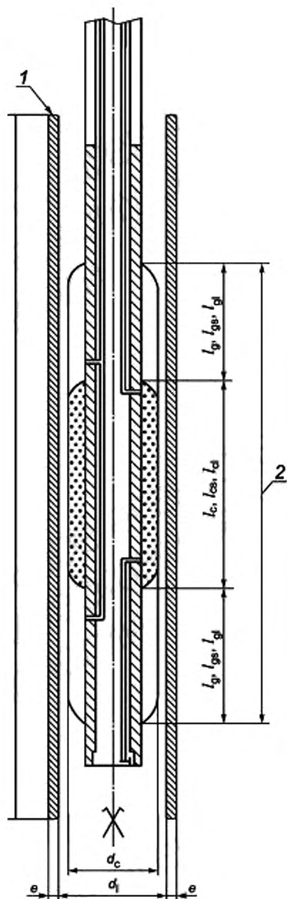
1 — тарировочный цилиндр, 2 — пьезометрический зонд
