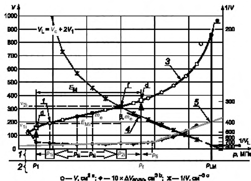
1 — начальная оценка; 2 — конечная проверка; 3 — двойная гиперболическая аппроксимирующая кривая; 4 — обратная прямая объема, соответствующая последним трем значениям; 5 — пример соответствия точек ползучести; i — начальный
