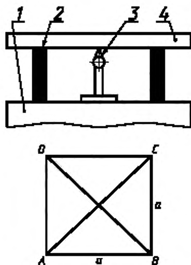
1 — плита; 2 — равновысокие опоры; 3 — индикатор; 4 — поверочная линейка
