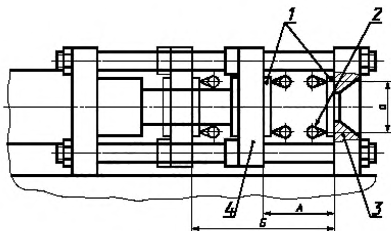
1 — проверочные линейки; 2 — нутромер; 3 — неподвижная плита; 4 — подвижная плита
