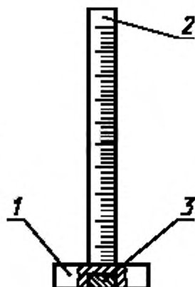
1 — основание; 2 — измерительная металлическая линейка; 3 — магнитный держатель
