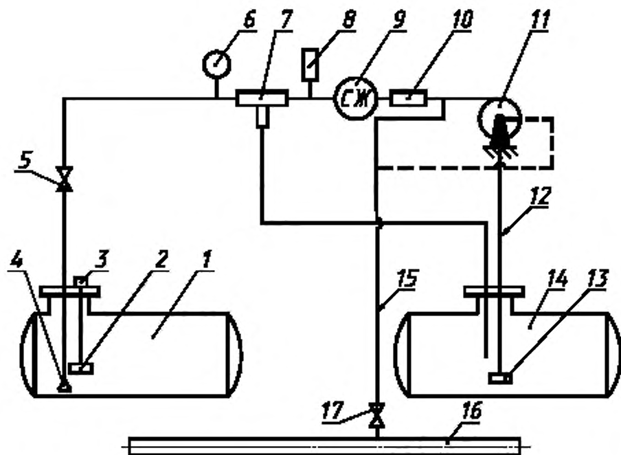
1 — поверяемый резервуар; 2 — поплавковый уровень; 3 — уровень; 4 — расширитель струи; 5, 17 — вентили; 6 — манометр; 7 — трехходовой кран; 8 — термометр (измеритель температуры); 9 — счетчик жидкости; 10 — дроссель; 11 — насос; 12 — всасывающая линия насоса; 13 — фильтр; 14 — приемный резервуар; 15 — линия технологической обвязки; 16 — технологический трубопровод (водопровод)
