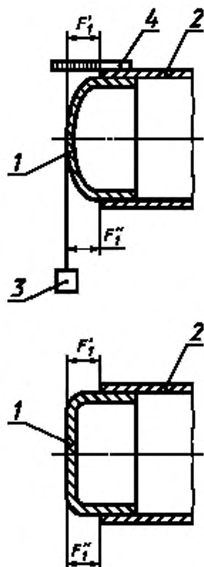
1 — днище; 2 — пояс; 3 — отвес; 4 — измерительная металлическая линейка
