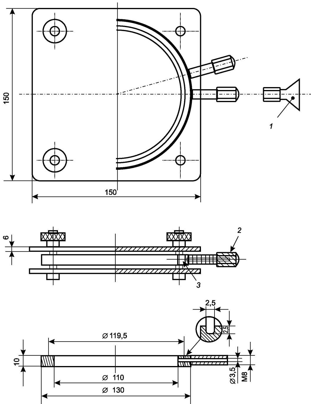
Рисунок С.4 – Камера, тип В
