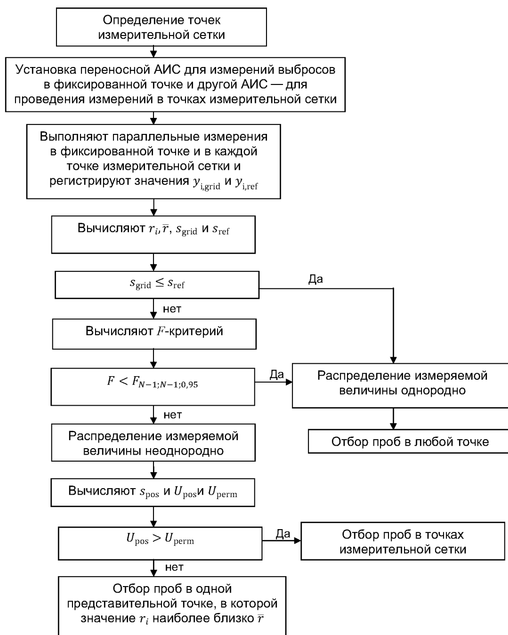
Рисунок 5 — Схема методики определения однородности
