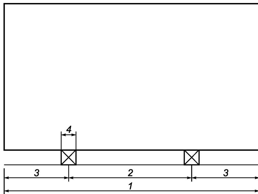
Рисунок 7 — Определение общего и локального отклонений от плоскостности
