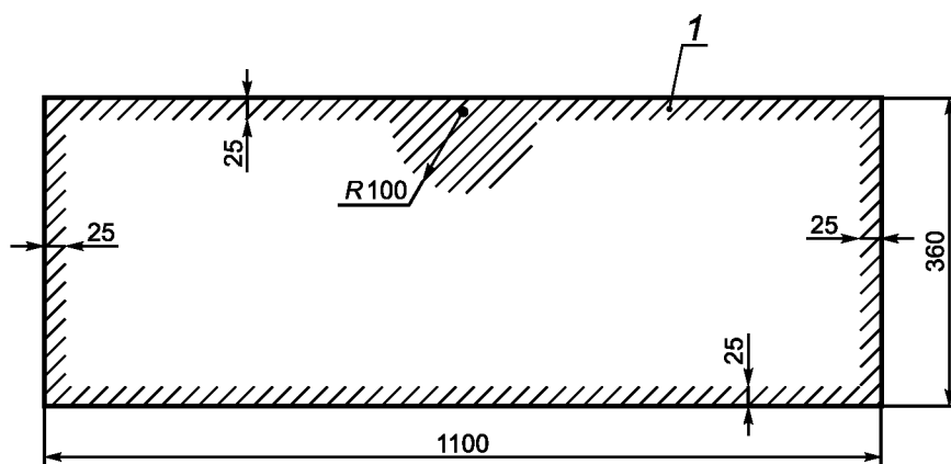
1 — область стекла, исключаемая из оценки результатов
