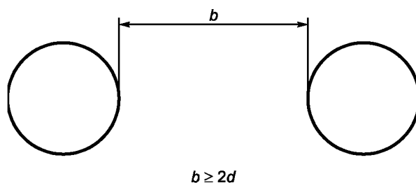
Рисунок 14 — Расстояние между кромками двух отверстий
