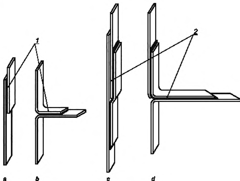
а — образец на сдвиг клеевого соединения анахлест гибких полимерных композитов, выполненного соединением липкой лентой; б — Т-образный образец на расслаивание клеевого соединения гибких полимерных композитов, выполненного соединением липкой лентой; в — образец на сдвиг клеевого соединения анахлест гибких полимерных композитов, выполненного нашовным клеевым соединением; д — Т-образный образец на расслаивание клеевого соединения гибких полимерных композитов, выполненного нашовным клеевым соединением; 1 — липкая лента; 2 — нашовная липкая лента
