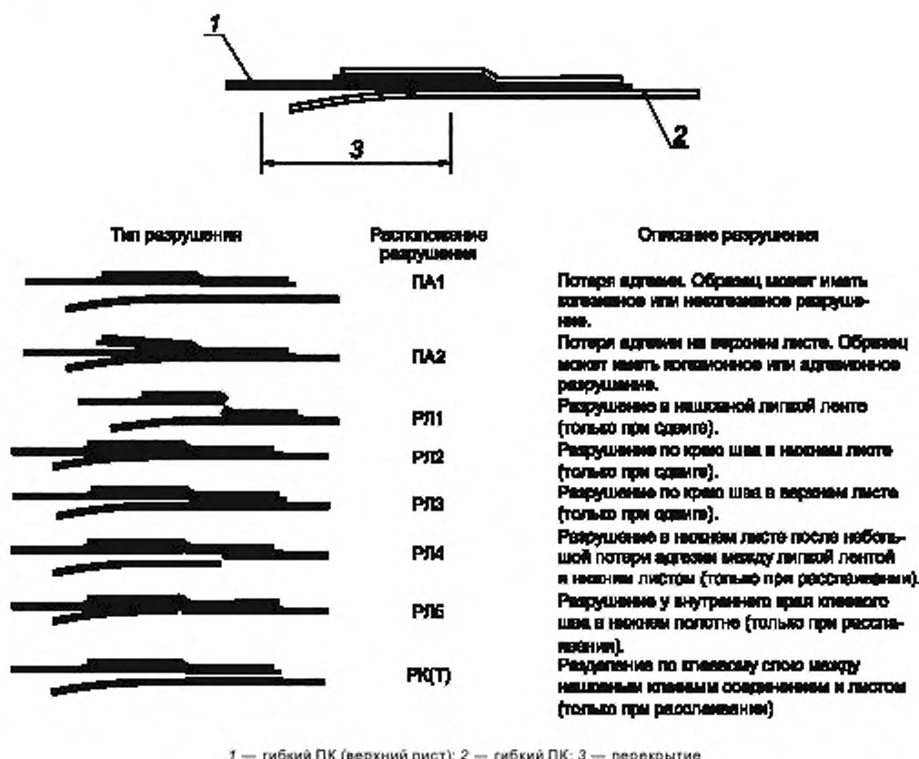
Рисунок 4 — Типы и расположения разрушений для образцов клеевого соединения внахлест, выполненного нашивным клеевым соединением
