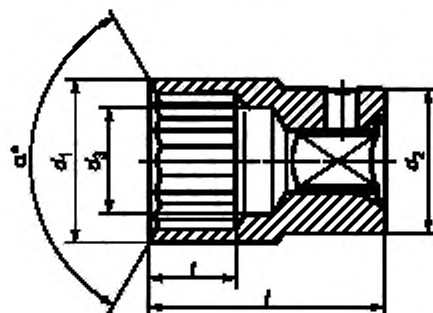
Рисунок 2 — Сменные головки с d_1 = d_2
