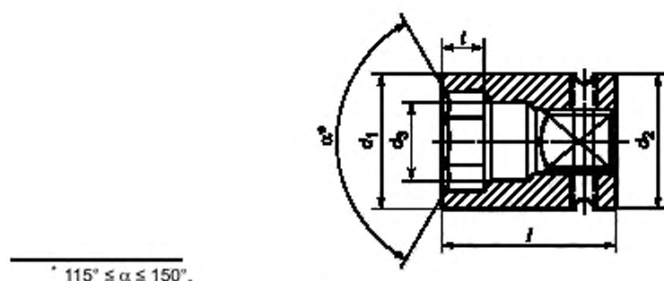
Рисунок 5 — Сменные головки с d_1 = d_2
