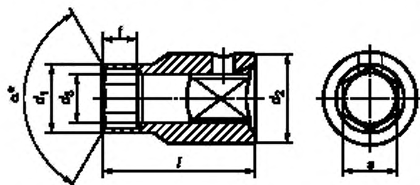
Рисунок 1 — Сменные головки с d_1 < d_2
