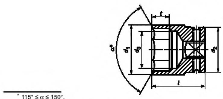
Рисунок 6 — Сменные головки с d_1 > d_2
