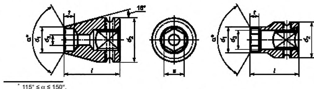
Рисунок 4 — Сменные головки с d_1 < d_2
