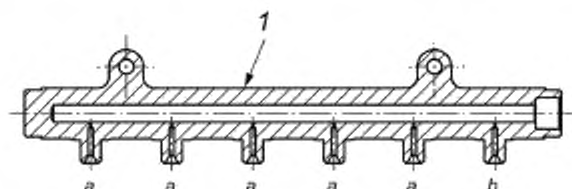
1 — аккумулятор для испытаний; a — выходные штуцера к форсункам; b — входной штуцер со стороны насоса высокого давления
