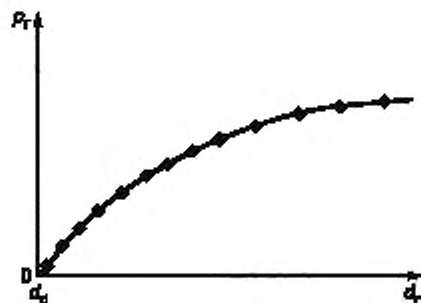
Рисунок А.1 — Кривая жесткости мембраны для гибкого дилатометра
