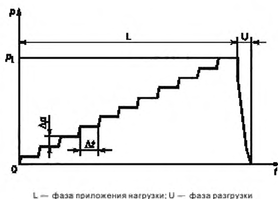
Рисунок В.3 — Пример программы испытания с приложением нагрузки (процедура С)
