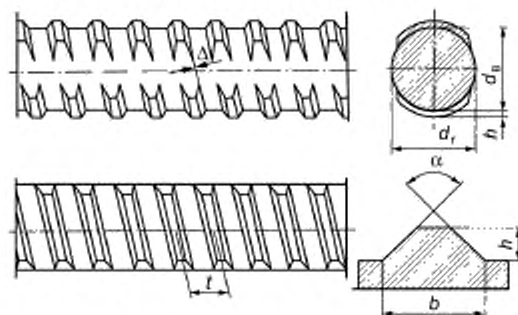
\Delta — величина отклонения винтовых выступов; d_g — максимальный диаметр винта без винтовых выступов; d_r — минимальный диаметр винта; h — высота поперечного ребра винтового выступа; f — шаг поперечного ребра; \alpha — угол наклона боковой поверхности поперечного ребра, град
