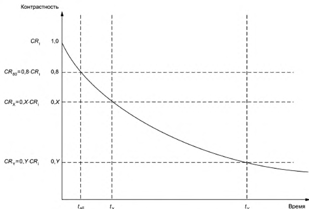
Рисунок 10 — Временные характеристики контрастности
