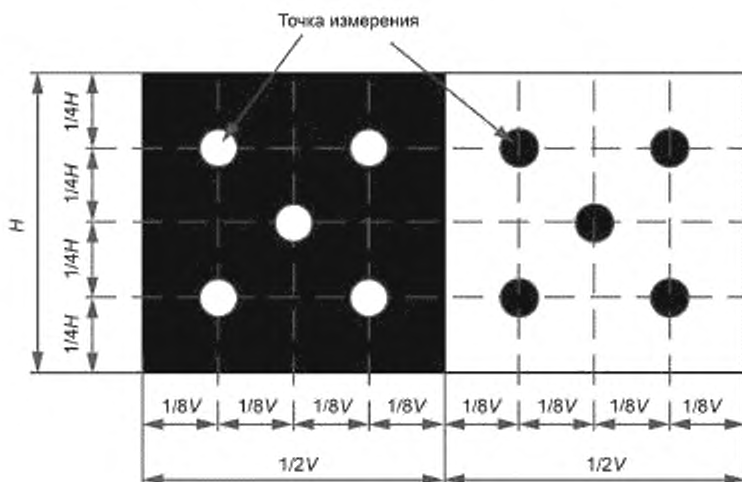
Рисунок 3 — Точки измерения
