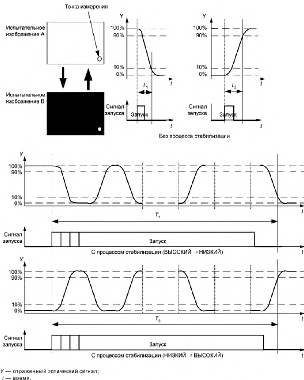
Рисунок 7 — Пример сигнала запуска и времени кадрового отклика (матричный дисплей)
