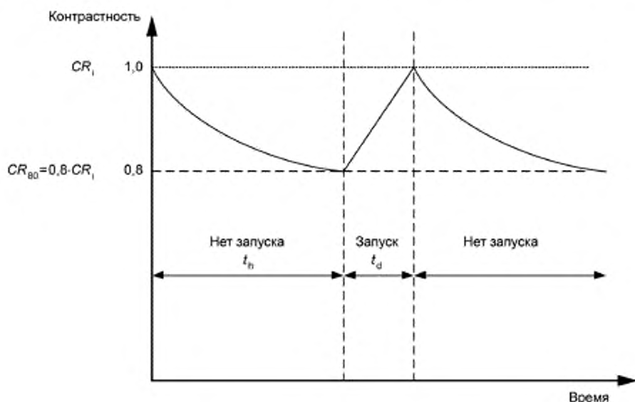
Рисунок 11 — Контрастность изображения и режим запуска
