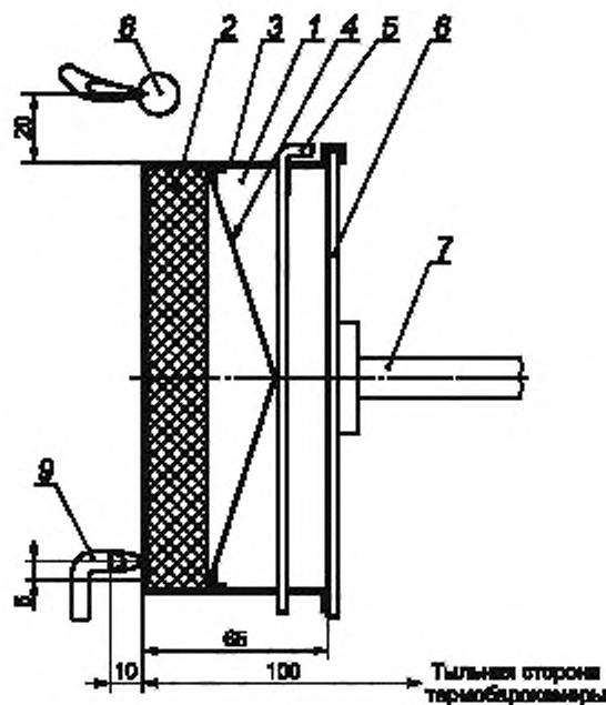
1 — держатель образца; 2 — образец; 3 — фиксирующая рамка; 4 — прижимная пружина; 5 — стопорный стержень; 6 — монтажная опора; 7 — подвижной стержень; 8 — верхняя запальная горелка; 9 — нижняя запальная горелка
