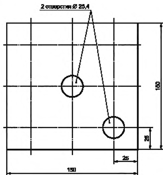
Рисунок А.8 — Панель для установки датчиков теплового потока
