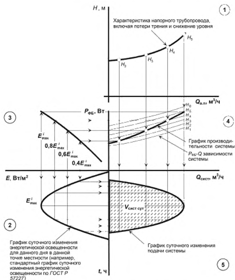
Рисунок 4 — Пример номограммы выходных характеристик автономной фотозлектрической насосной системы для подачи воды (система с центробежным насосом, тип А)
