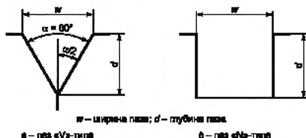
Рисунок 1 — Типы настроечных пазов
