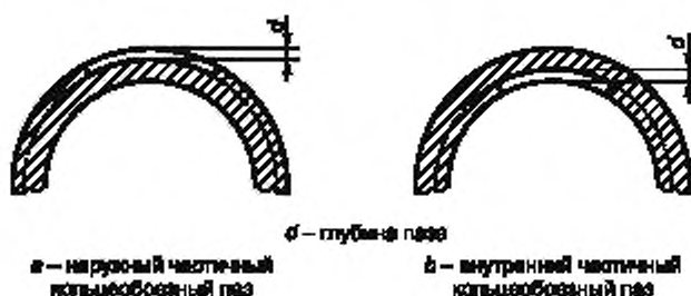
Рисунок 2 — Поперечный настроечный паз
