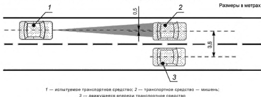
Рисунок 13 — Испытание на обнаружение (начальные условия)
