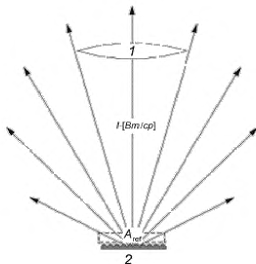
1 — приемное устройство; 2 — отражатель
