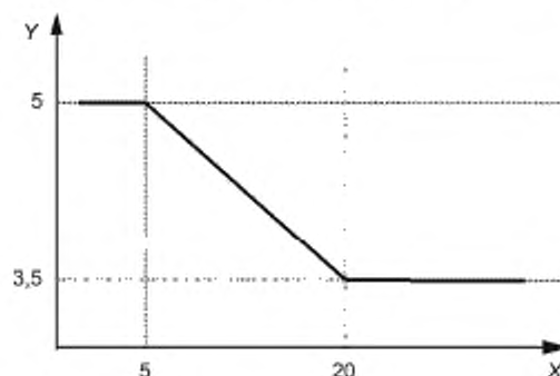
Рисунок 7 — Максимальное замедление
