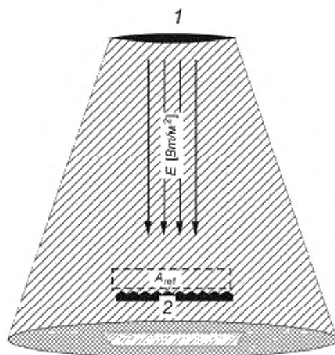
1 — излучатель; 2 — отражатель
