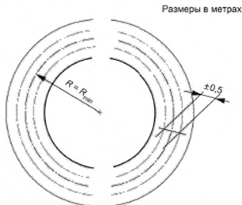
Рисунок 15 — Схема испытательного трека
