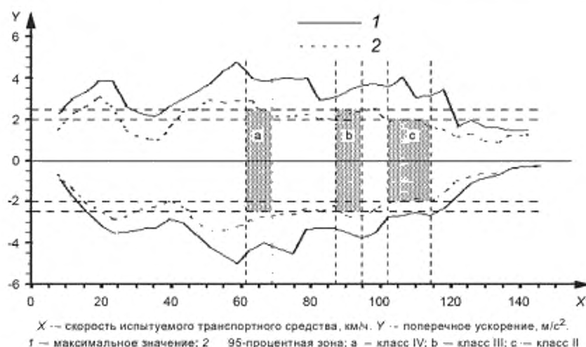
Рисунок 6 — Поперечное ускорение для среднего водителя
