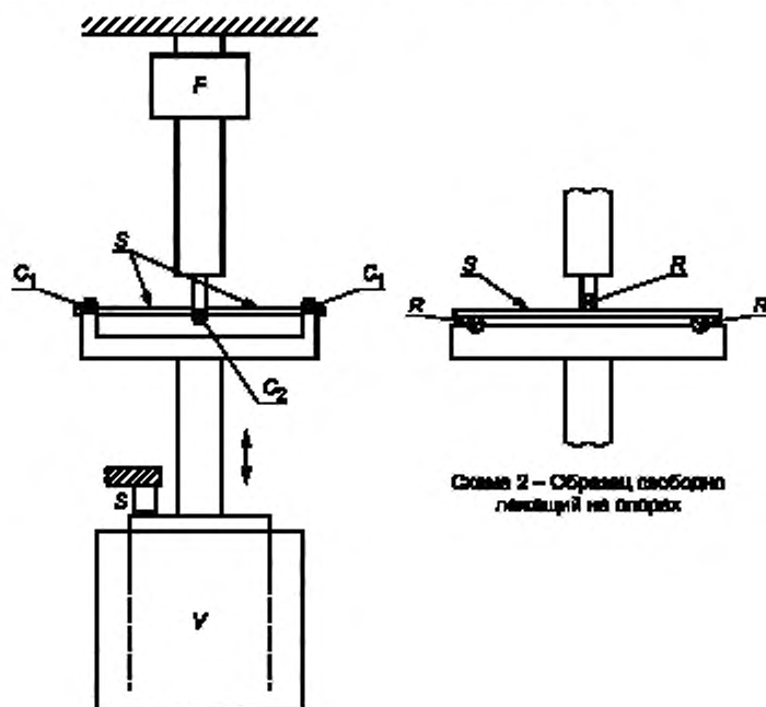
Схема 1 — Зажимный образец
