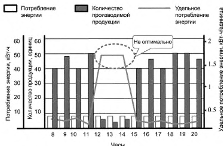
Рисунок Е.4 — Диаграмма тенденций удельного потребления энергии
