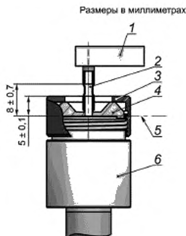
1 — слуховой аппарат (модульного типа); 2 — гибкая соединительная трубка, обычно с внутренним диаметром 2 мм; 3 — фиксирующий фланец (хомут); 4 — трубчатое соединительное устройство, обычно с внутренним диаметром 2 мм; 5 — опорная плоскость; 6 — имитатор внутреннего уха
