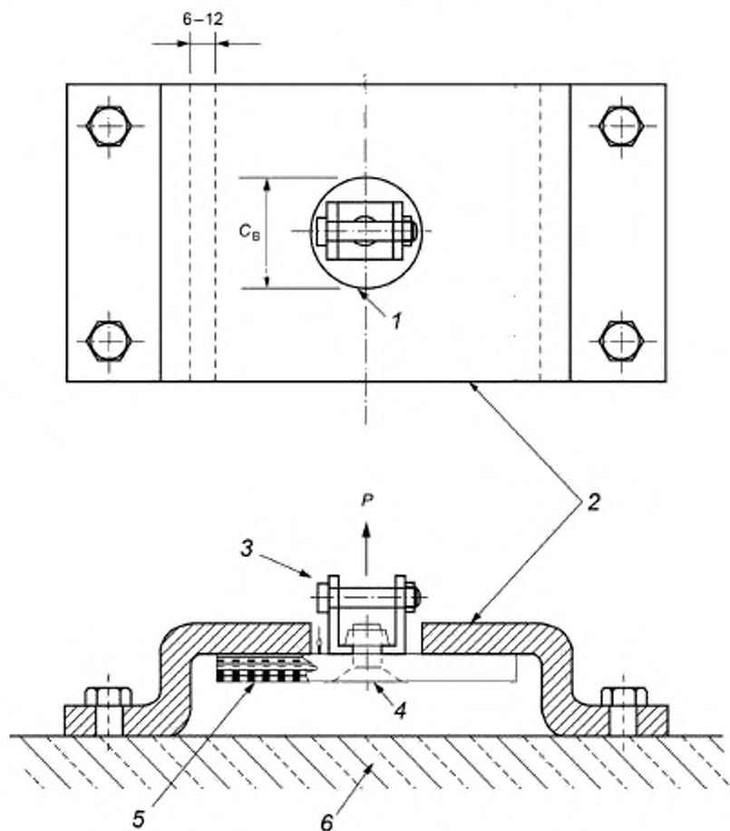
C_{\text{в}} — диаметр отверстия в швеллере; P — нагрузка; 1 — отверстие в швеллере; 2 — швеллер; 3 — крестовина, 4 — установленный болт; 5 — образец; 6 — плита основания
