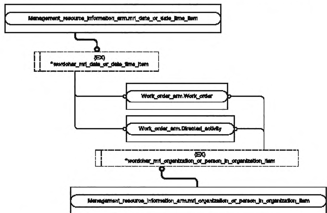
Рисунок С.4 — Представление ПЭМ на уровне объектов в формате EXPRESS-G. Диаграмма 3 из 4
