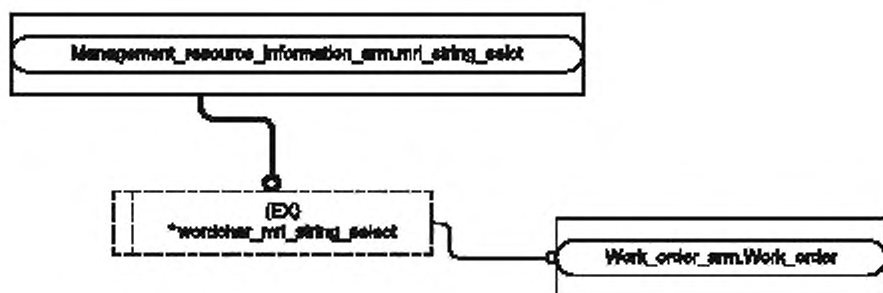
Рисунок С.5 — Представление ПЗМ на уровне объектов в формате EXPRESS-G. Диаграмма 4 из 4
