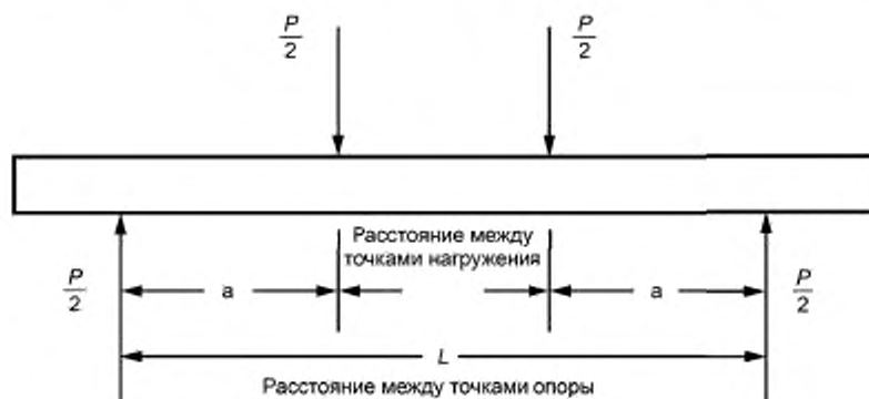
Рисунок X1.1 — Схема нагружения в случае расстояния между точками нагружения, не равного одной трети расстояния между опорами
