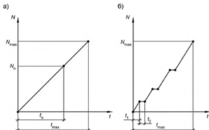
Рисунок 1 — Диаграмма нагружения конструкции непрерывно возрастающей (а) и ступенчатой (б) нагрузками
