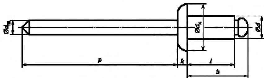
Рисунок 1 — Размеры заклепок
