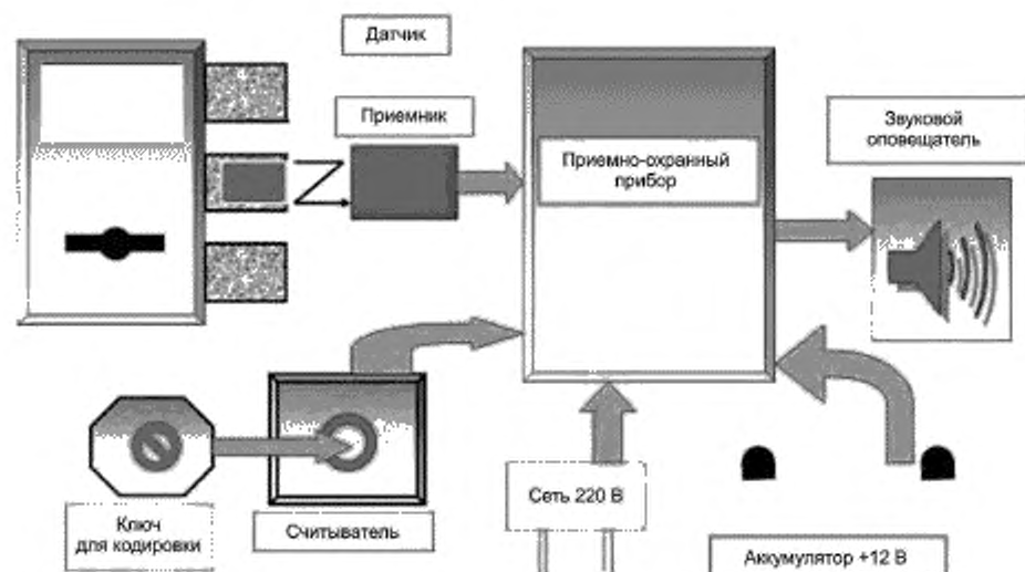
Рисунок Г.1 — Блок-схема системы раннего реагирования
