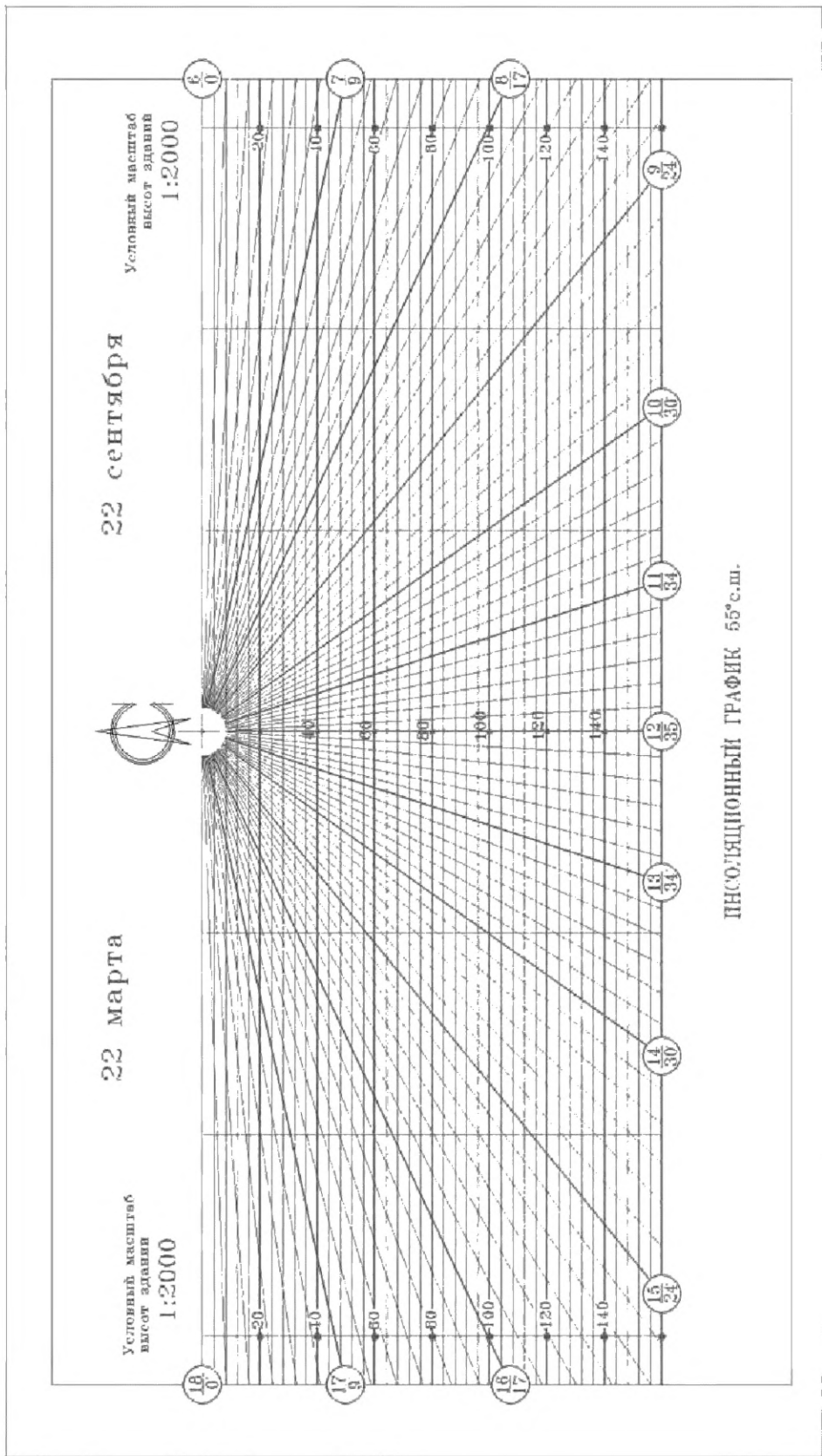
Рисунок В.17 — Инсоляционный график для города Москвы (55° с. ш.) в масштабе 1:2000
