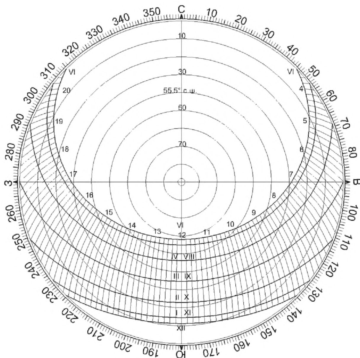
Рисунок Г.14 — Солнечная карта с равнопромежуточными альмукантаратами для города Москвы на 55,5^\circ с. ш.
