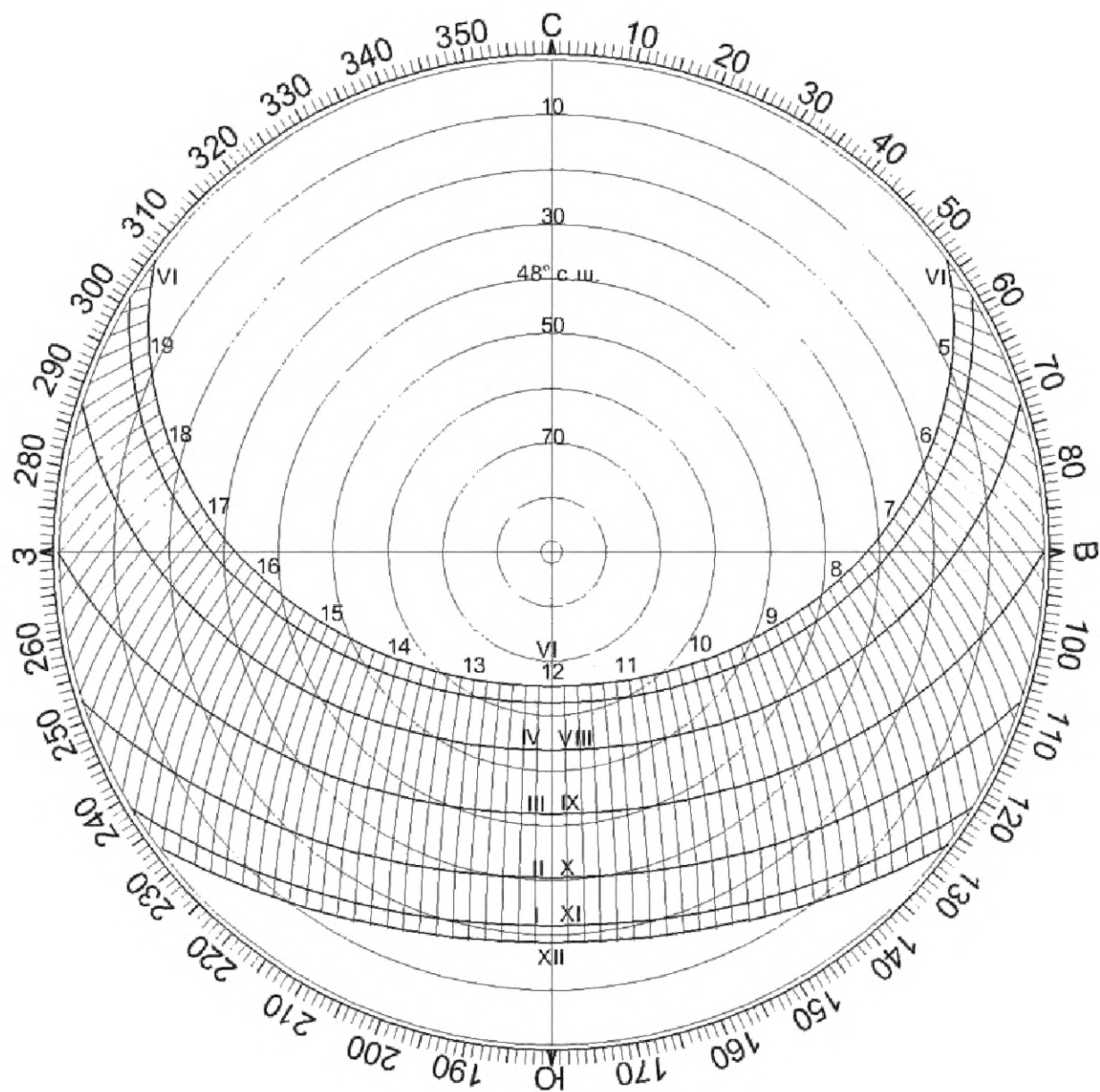
Рисунок Г.5 — Солнечная карта с равнопромежуточными альмукантаратами для территории Российской Федерации, расположенной на 48° с. ш.
