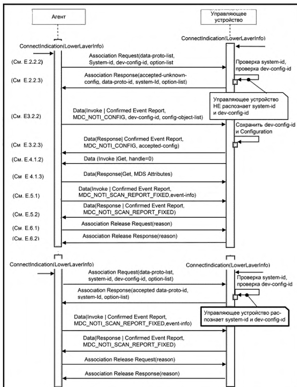
Рисунок D.1 — Диаграмма последовательности сообщений для приведенного примера использования пневматометра
