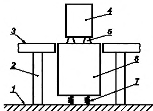
1 — грунтовое основание; 2 — стойка; 3 — пол лаборатории; 4 — испытуемое оборудование а ; 5 — жесткие опоры для установки испытуемого оборудования на фундамент б ; 6 — жесткий и массивный испытательный стенд с ; 7 — упругое опирание испытательного стенда на грунтовое основание д
