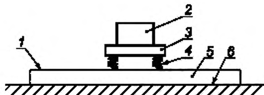
1 — пол лаборатории; 2 — испытуемое оборудование а ; 3 — крепёжное приспособление б ; 4 — упругие опоры крепёжного приспособления (практически свободный подвес) в ; 5 — фундамент г ; 6 — грунтовое основание
