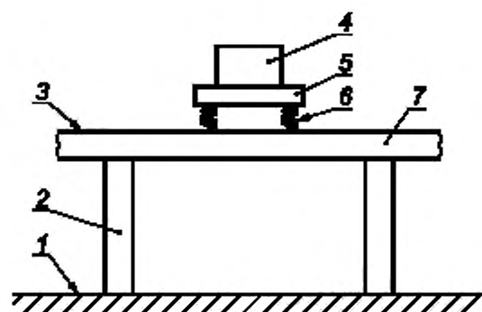
1 — грунтовое основание; 2 — стойка; 3 — пол лаборатории; 4 — испытуемое оборудование а ; 5 — крепежное приспособление; 6 — упругие опоры для установки испытуемого оборудования на фундамент б ; 7 — фундамент с
