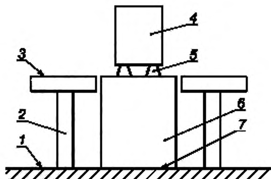
1 — грунтовое основание; 2 — стойка; 3 — пол лаборатории; 4 — испытуемое оборудование а ; 5 — жесткие опоры для установки испытуемого оборудования на фундамент (см. 4.7.2.3); 6 — жесткий и массивный испытательный стенд (см. 4.7.2.1); 7 — жесткое опирание испытательного стенда на грунтовое основание
