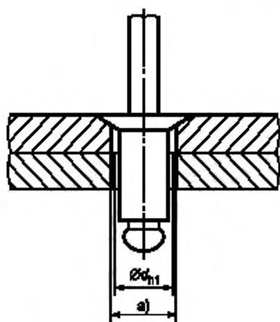
а) Увеличенное отверстие с зазором.
