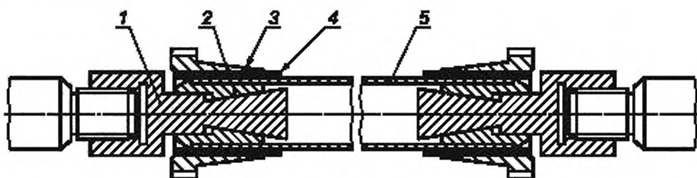
1 — шпилька; 2 — сегментированные захваты; 3 — втулка; 4 — укрепляющий пояс; 5 — образец для испытания
