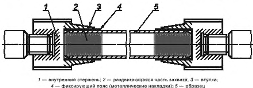
Рисунок А.1 — Захват для крепления образца с внутренним стержнем
