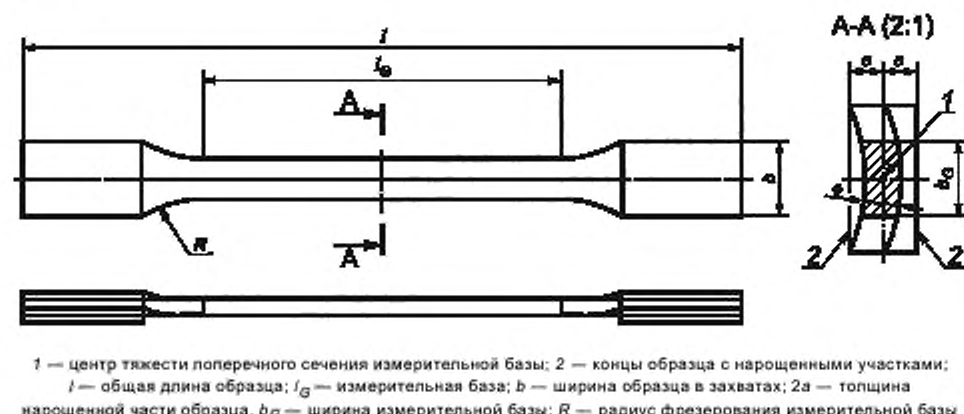
Рисунок 2 — Образец в форме лопатки (для метода А)
