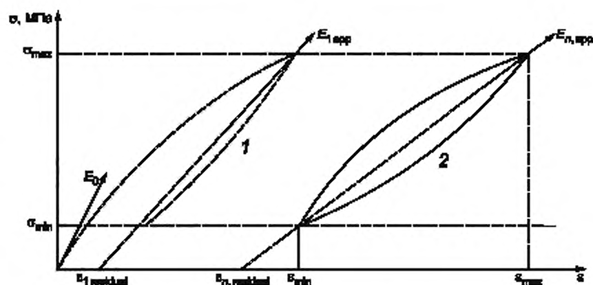
1 — первый цикл нагружения; 2 — n-й цикл нагружения
