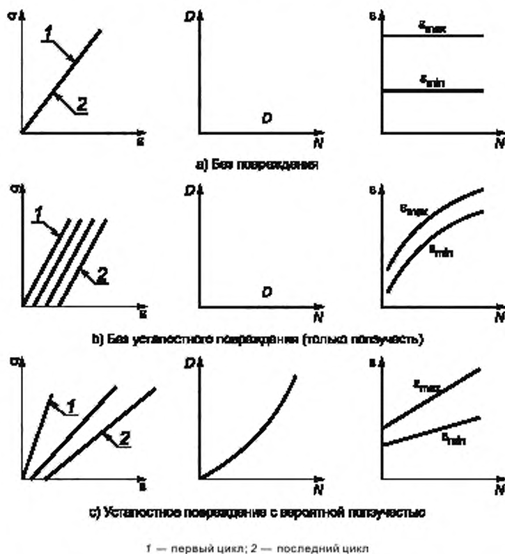
Рисунок А.1 — Схематическое развитие Е: а) без повреждения, б) ползучесть, без усталостного повреждения, и с) усталостное повреждение с вероятной ползучестью
