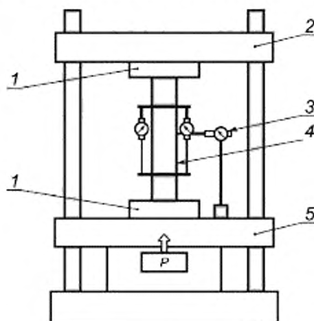
1 — нагрузочная площадка, 2 — верхняя траверса; 3 — прибор для регистрации деформаций; 4 — образец, 5 — основание испытательной машины; P — нагрузка
