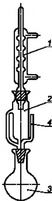
1 — холодильник; 2 — экстрактор; 3 — экстракционная колба; 4 — сифонная трубка
