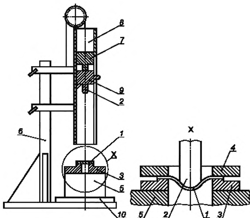
1 — образец для испытания; 2 — полусферический наконечник бойка; 3 — опора образца для испытаний (опорное кольцо); 4 — зажимное кольцо; 5 — основание; 6 — стойка для системы свободно падающего груза; 7 — система удержания и размыкания для нагруженного бойка; 8 — направляющий вал для нагруженного бойка; 9 — нагруженный боек; 10 — акустическая изоляция (дополнительная опция)
