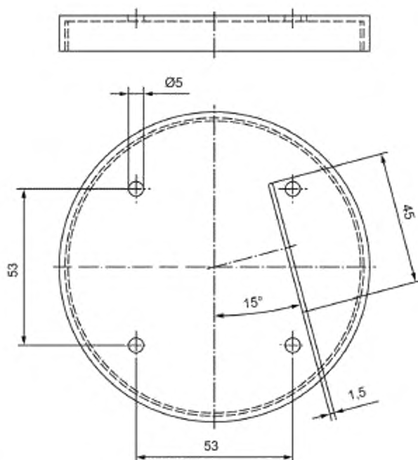
Рисунок В.5 — Часть 5: сосуд с закручивающейся крышкой (на чертеже приведена только крышка)
