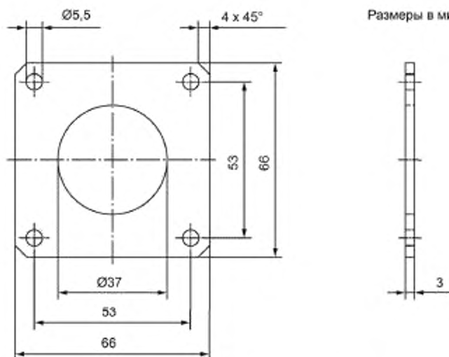
Рисунок В.2 — Часть 2: крепежный обруч
