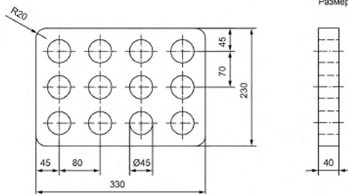
Рисунок В.4 — Часть 4: плавающая платформа с отверстиями
