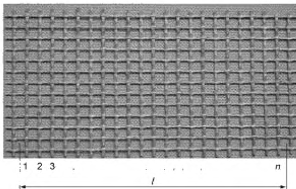
l — измеряемое расстояние от середины ячейки стеклосетки до середины ячейки стеклосетки
