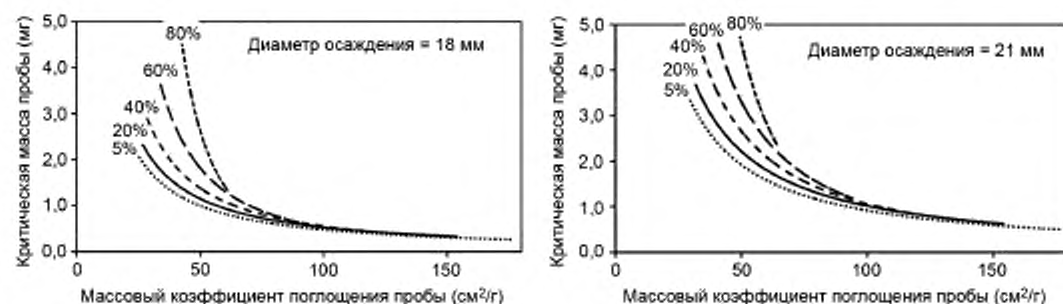
Рисунок С.1 — Критическая масса пробы, которая приводит к приурочению определенной концентрации кварца на 10 % для широкого диапазона массового коэффициента поглощения пробы (излучение меди). В смеси присутствует 5 % кварца
