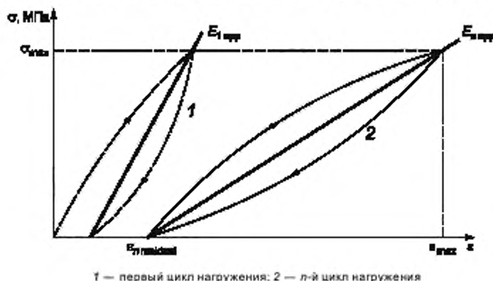
Рисунок 2 — Отнулевой цикл нагружения
