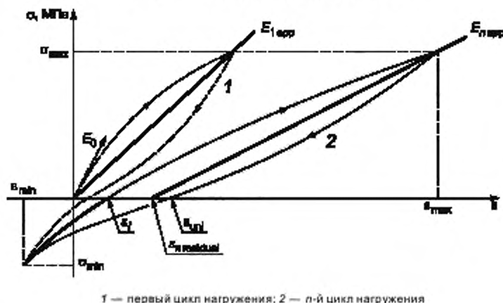
Рисунок 3 — Знакопеременный цикл нагружения
