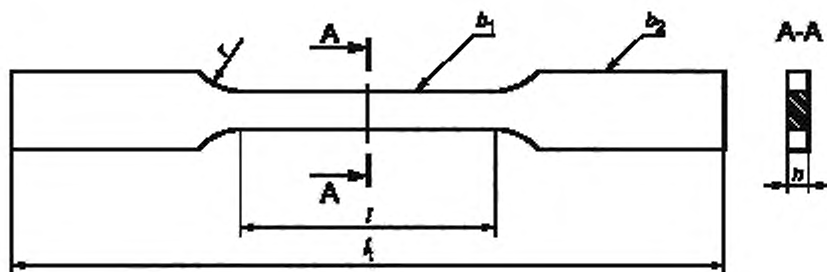
l — длина узкой параллельной части; l_0 — общая длина; h — толщина; b_1 — ширина в пределах измерительной базы; b_2 — ширина на концах; r — радиус
