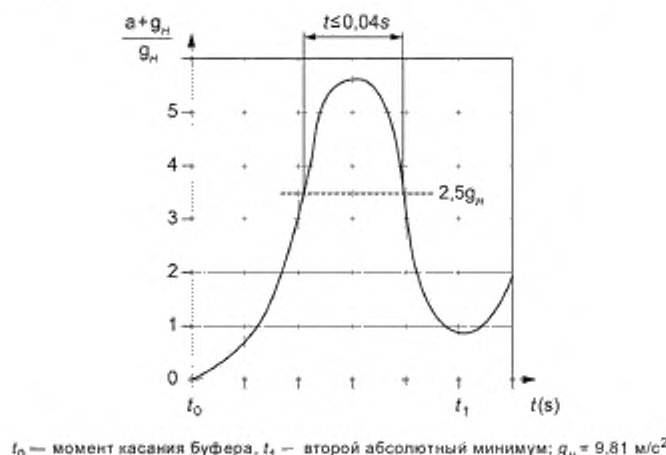
Рисунок А.1 — График торможения
