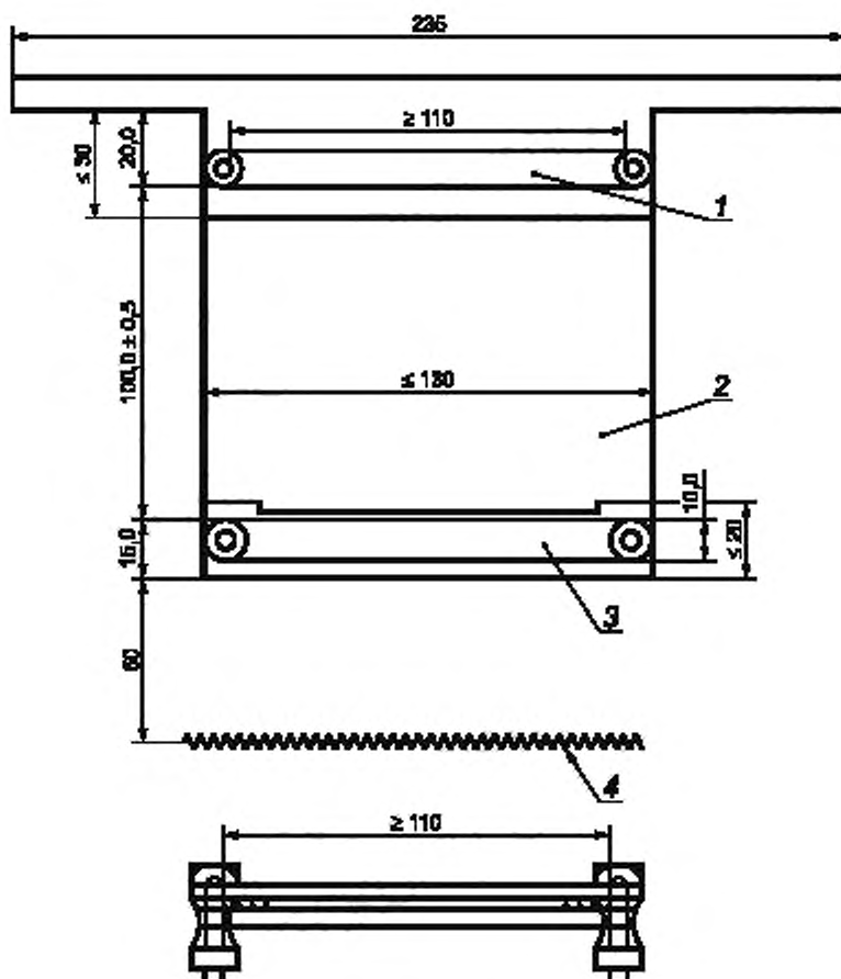
1 — верхний зажим, 2 — образец, 3 — нижний зажим; 4 — сито
