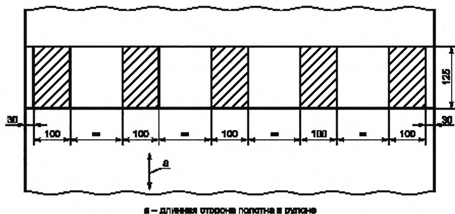
Рисунок 3 — Пример расположения образцов
