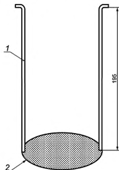
Рисунок 1 — Сито с подвеской
