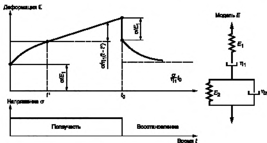
Рисунок Х6.3 — Четырехэлементная модель
