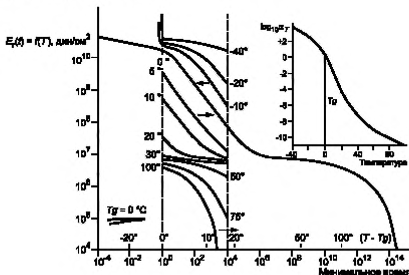
Рисунок Х5.2 — Обобщающая кривая снятия напряжения
