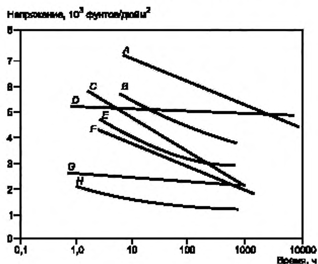
Рисунок X3.4 — Контур разрушения при ползучести
