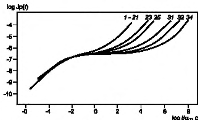
Рисунок X5.3 — Кривая податливости
