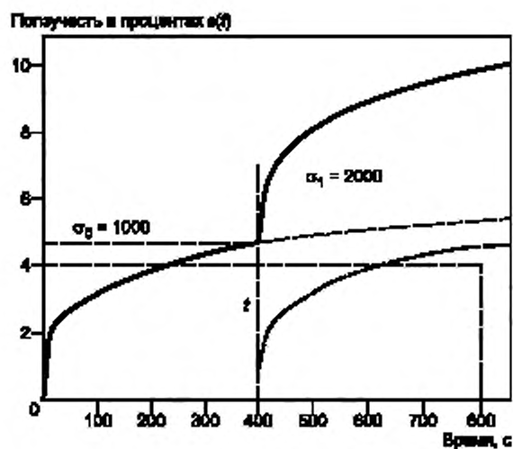
Рисунок X5.1 — Принцип Больцмана
