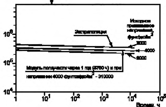
Рисунок 3 — Модуль ползучести 30% полибутилентерфалата, армированного стекловолокном, при 212° F, экстраполированный для получения расчетного модуля для точки 1 год
