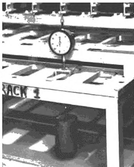
Рисунок 2 — Устройство для испытания на ползучесть при изгибе
