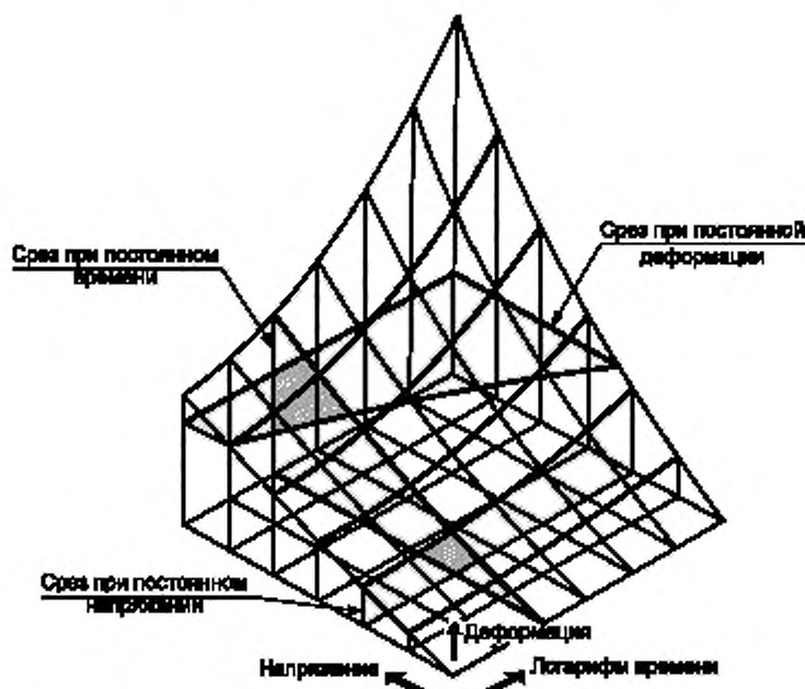
Рисунок Х4.1 — Постоянные координаты «напряжения—деформации—времени»
