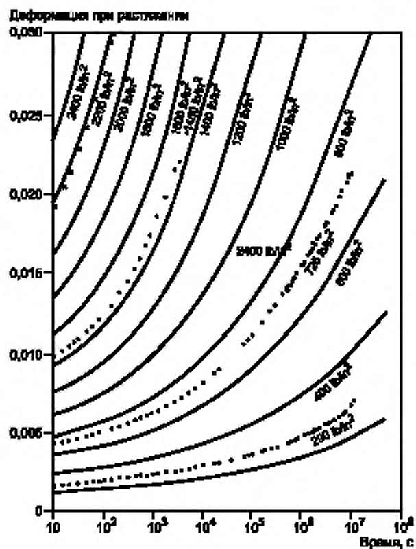
Рисунок X4.3 — Числовая интерполяция значений ползучести
