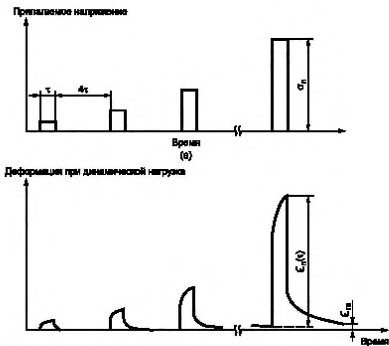
Рисунок X4.2 — Изохронные данные
