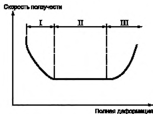
Рисунок X3.1 — Скорость ползучести
